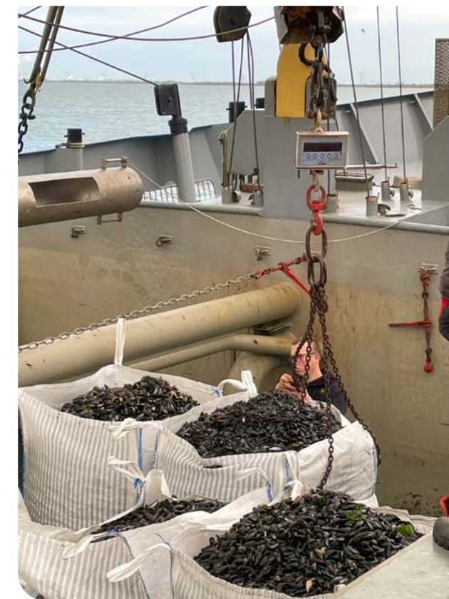
Het nieuwe weegsysteem zit tussen de kraan en de big bags.
